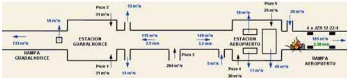
Figura 10. Esquema de resultados de simulación con ventiladores de chorro en Rampa Aeropuerto
