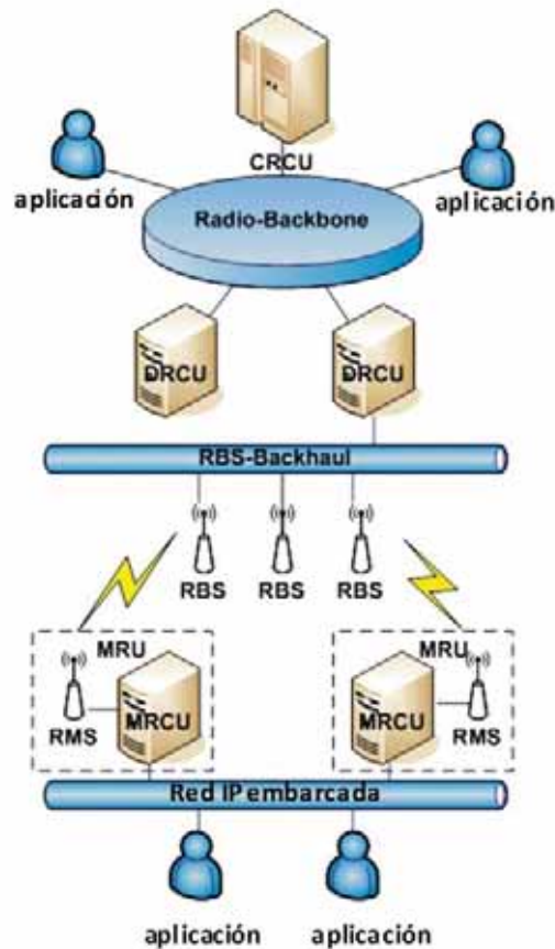
Figura 1: Arquitectura del sistema TRainCom® MT
